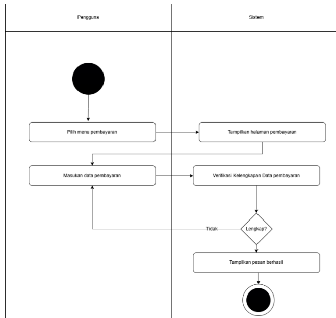
Gambar 4.10 Activity Diagram Tambah Pembayaran
