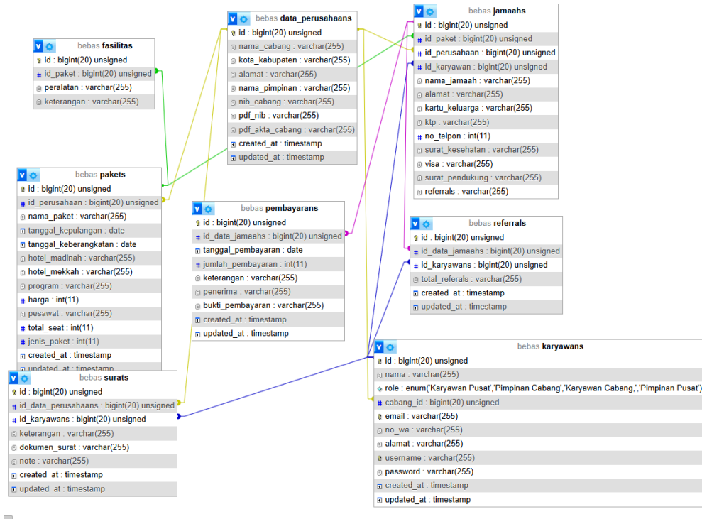
Gambar 4.35 Database dan Relasi antar Tabel
