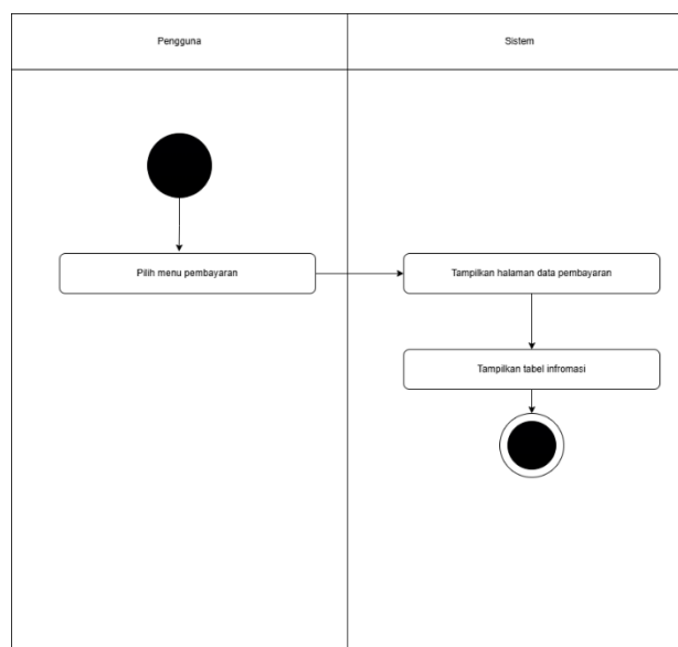
Gambar 4.13 Activity Diagram Lihat Pembayaran
