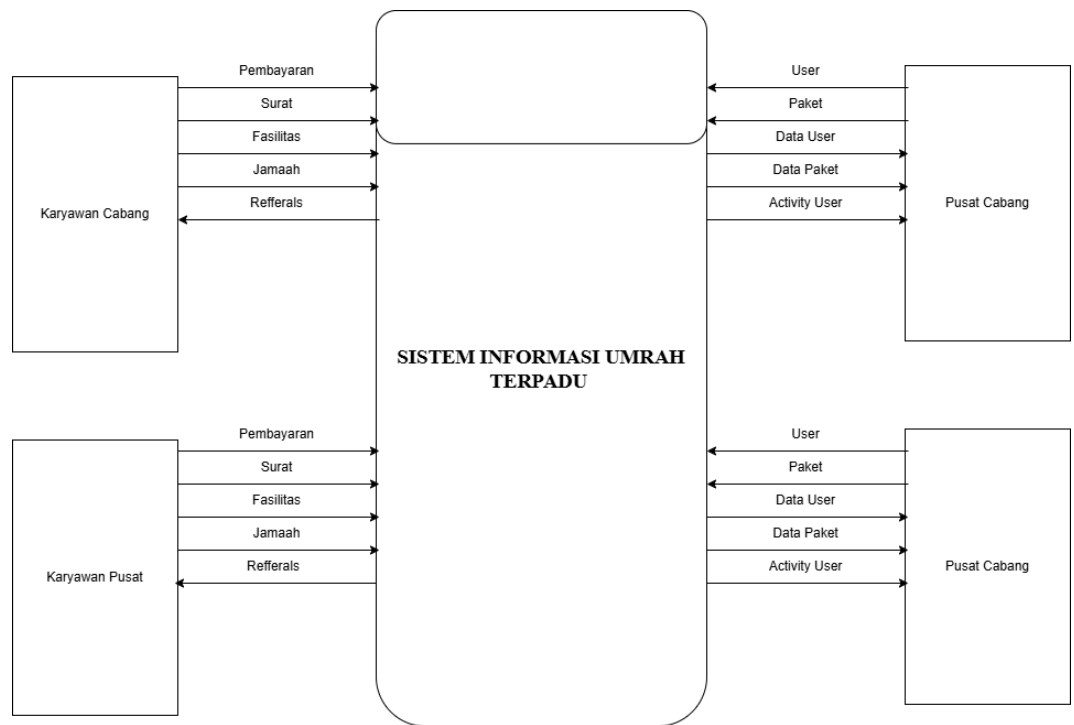
Gambar 4.28 Diagram Konteks
